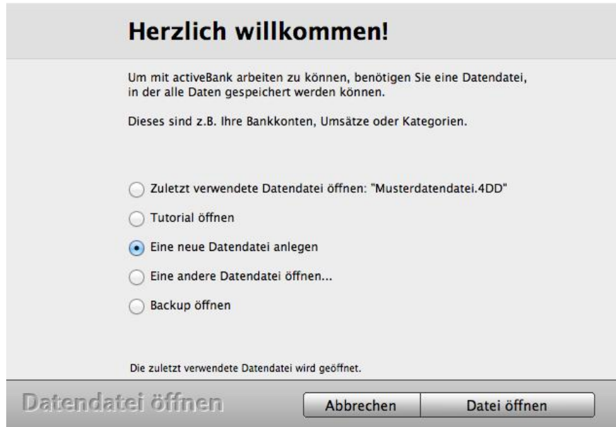
Datendatei-Auswahldialog
