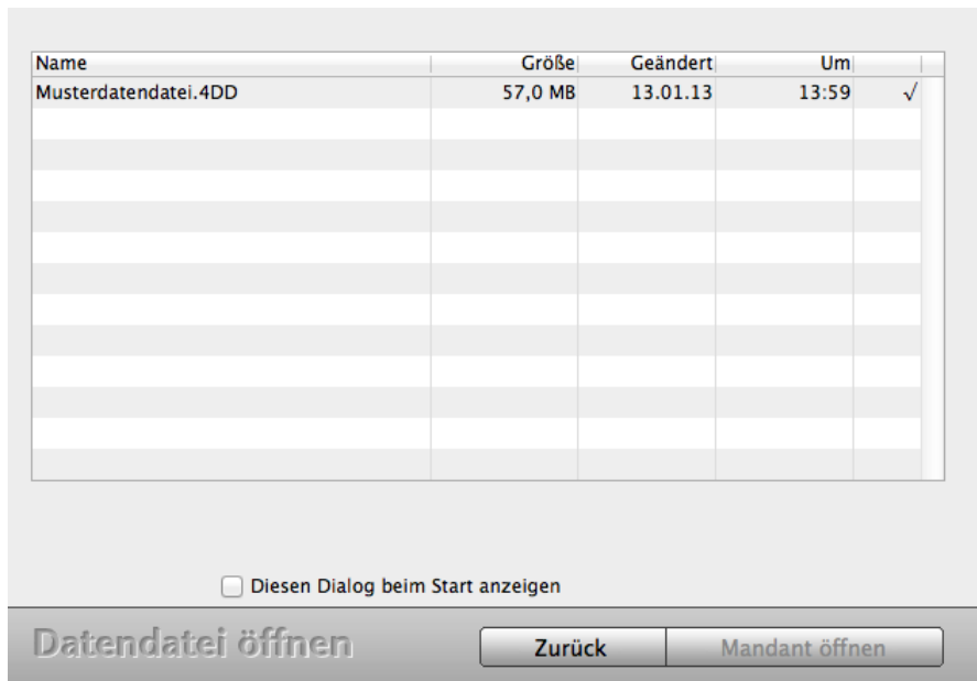
Datendatei öffnen-Auswahldialog
